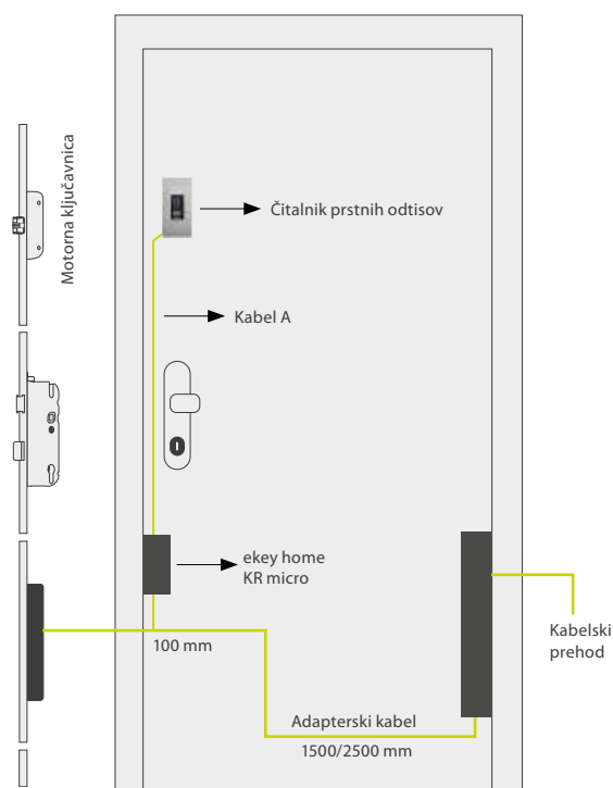
Konfiguracija "KLJ" - krmilnik micro pri ključavnici
