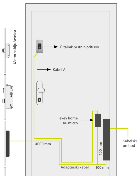
Konfiguracija "KAP" - krmilnik micro pri kabelskem prehodu
