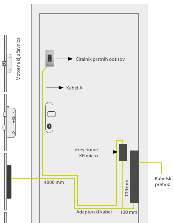
Konfiguracija "KAP" - krmilnik micro pri kablenskem prehodu
